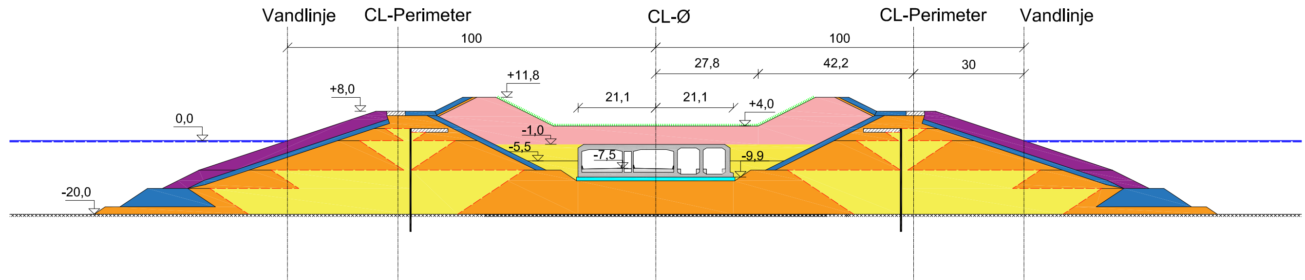
Snit B-B
